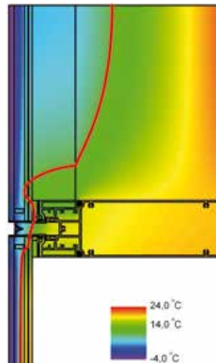
Energetische Überprüfung eines Fassadensystems durch Isothermenberechnungen
