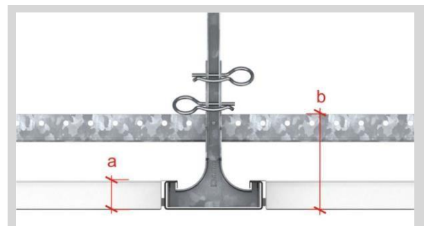
Поперечное сечение – потолочная панель тип 2
