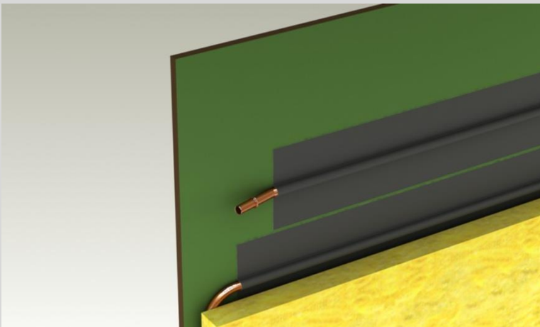
Schematische Darstellung - Wandpaneel Lindner Thermowall Typ 3
